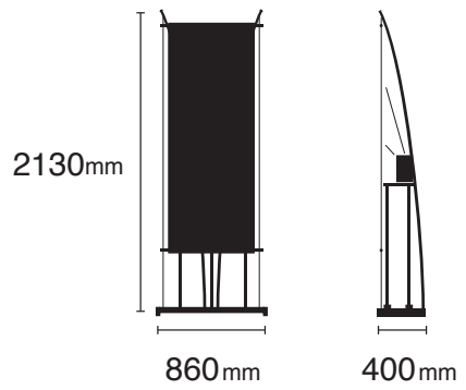
【組立寸法図】
